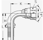
Фитинг 90° JIS (гайка) (внутренняя дюймовая резьба, внутренний конус 74°)
