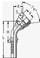
Фитинг 45° JIS (гайка) (внутренняя дюймовая резьба, внутренний конус 74°)
