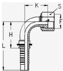
Фитинг 90° ORFS (гайка) (двойная резьба)
